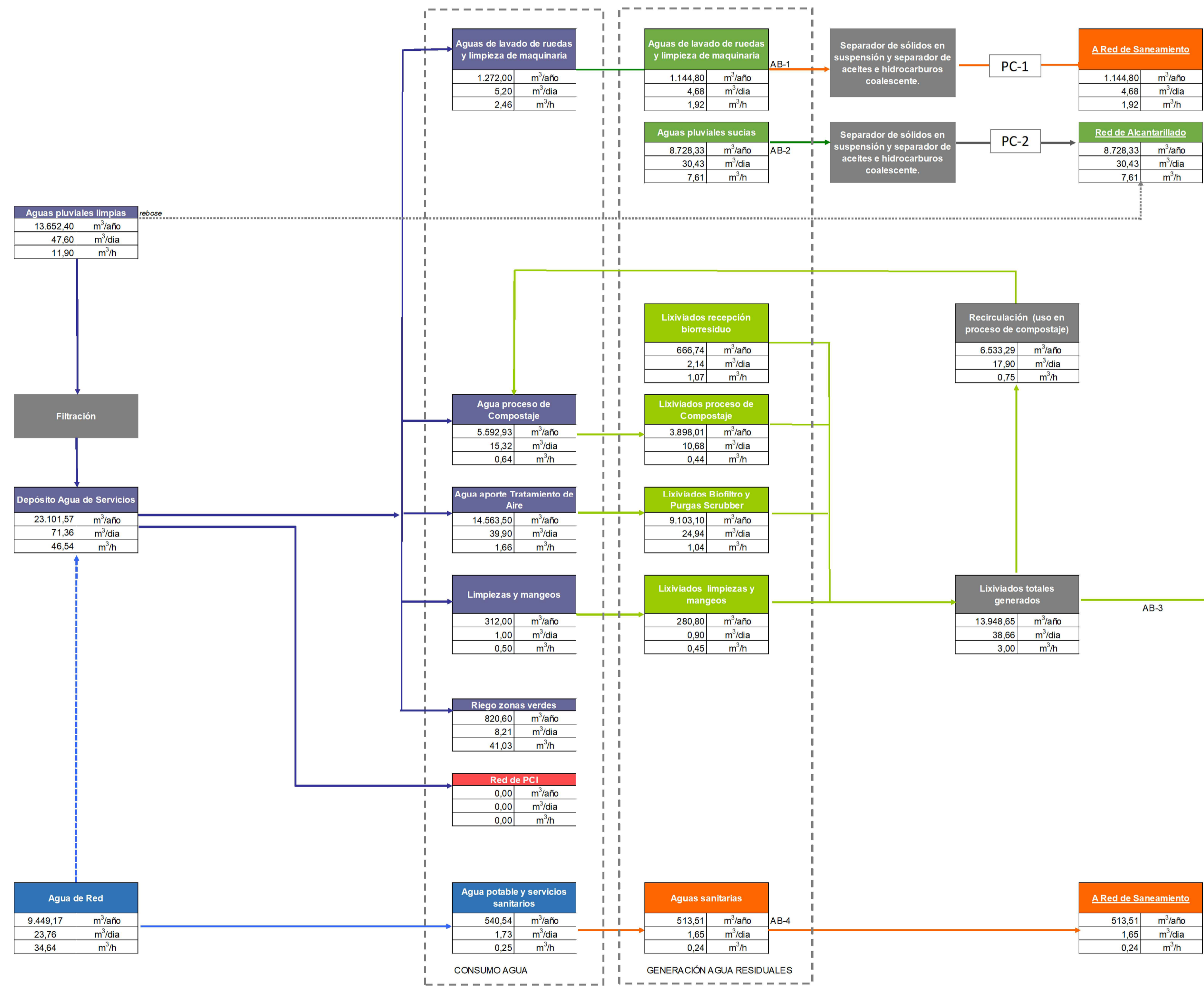
BALANCE DE AGUAS CAUDALES MÁXIMO FASE 1
