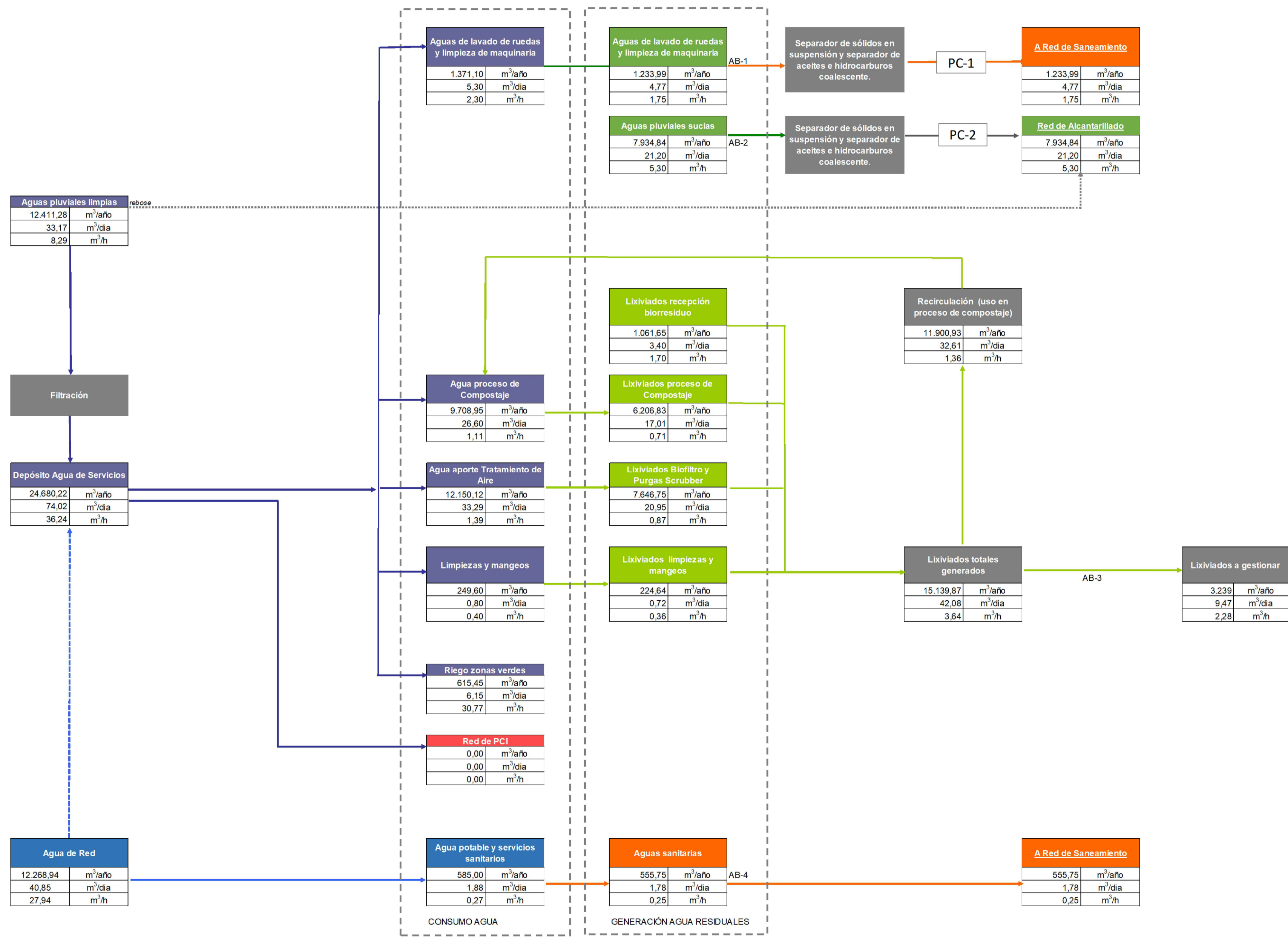
BALANCE DE AGUAS CAUDALES MEDIO FASE 2
