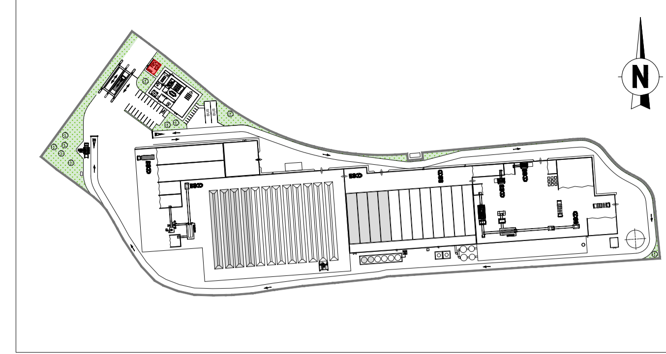
PLANTA LLAVE
