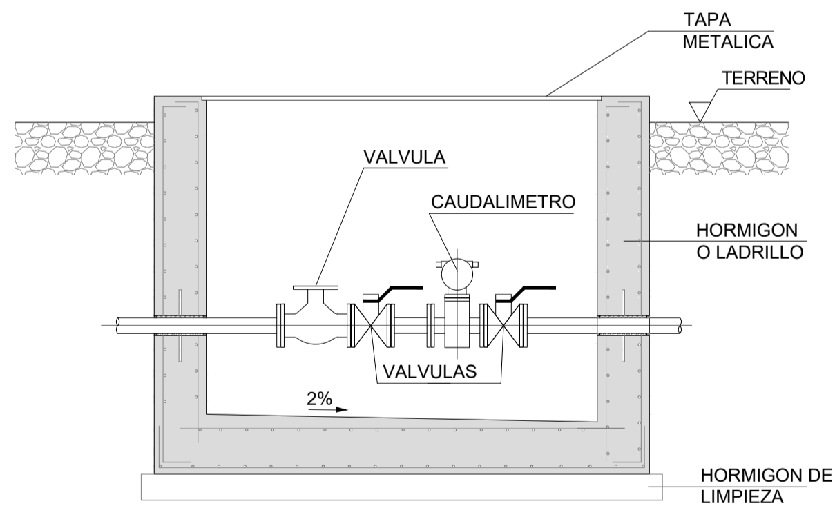
SECTION TIPO A-A ESCALA: S/E
