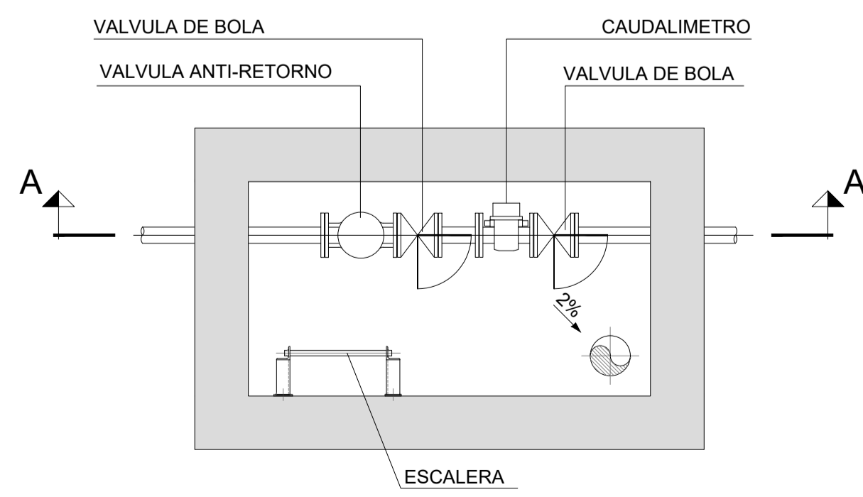
ARQUETA ACOMETIDA DETALLE TIPO ESCALA: S/E
