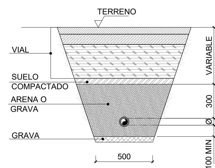
SECCION TIPO ESCALA: S/E
