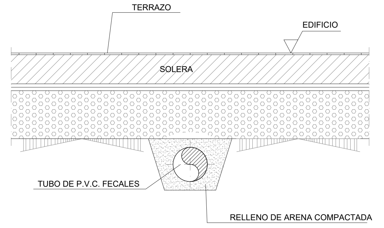
SECCION TIPO BAJO EDIFICIO ESCALA: S/E
