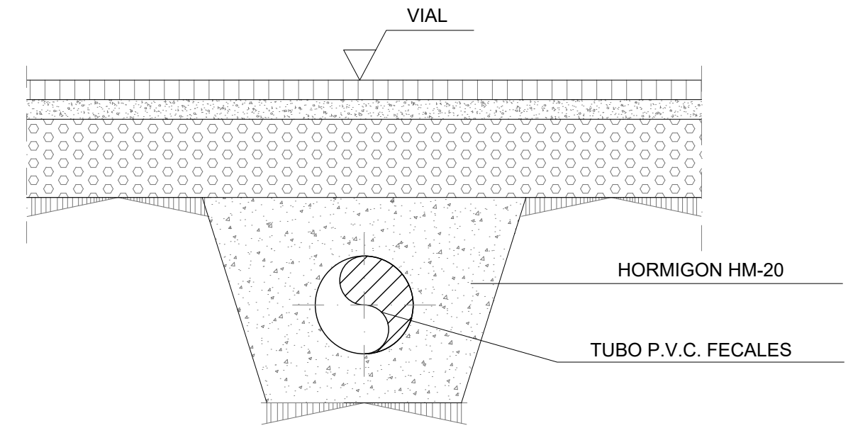
SECCION TIPO BAJO VIAL ESCALA: S/E
