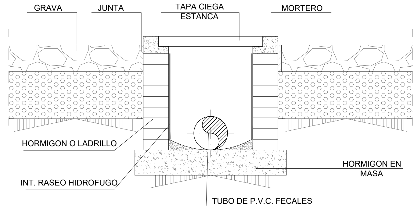
SECCION ARQUETA TIPO ESCALA: S/E
