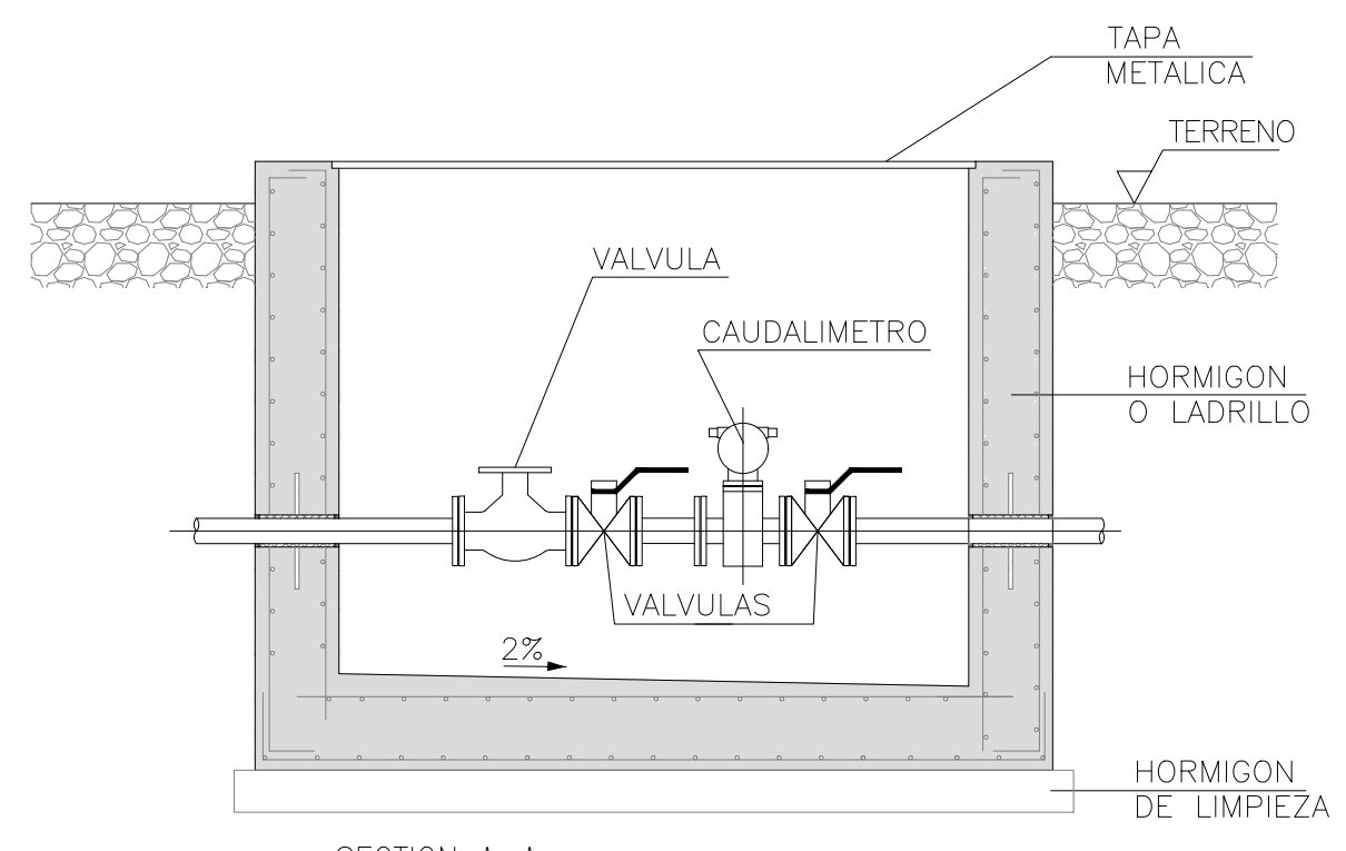
SECTION A-A ESCALA: S/E
