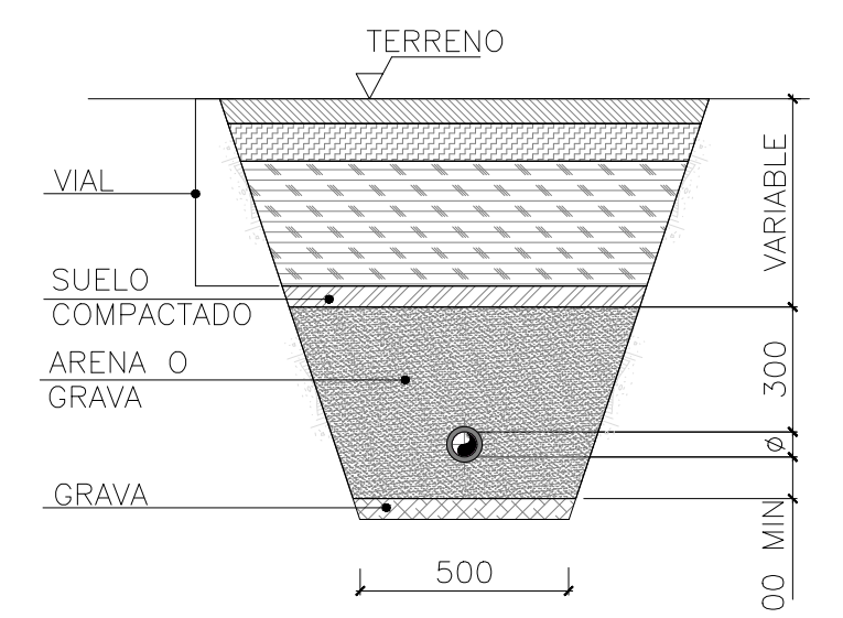
SECCION TIPO ESCALA: S/E
