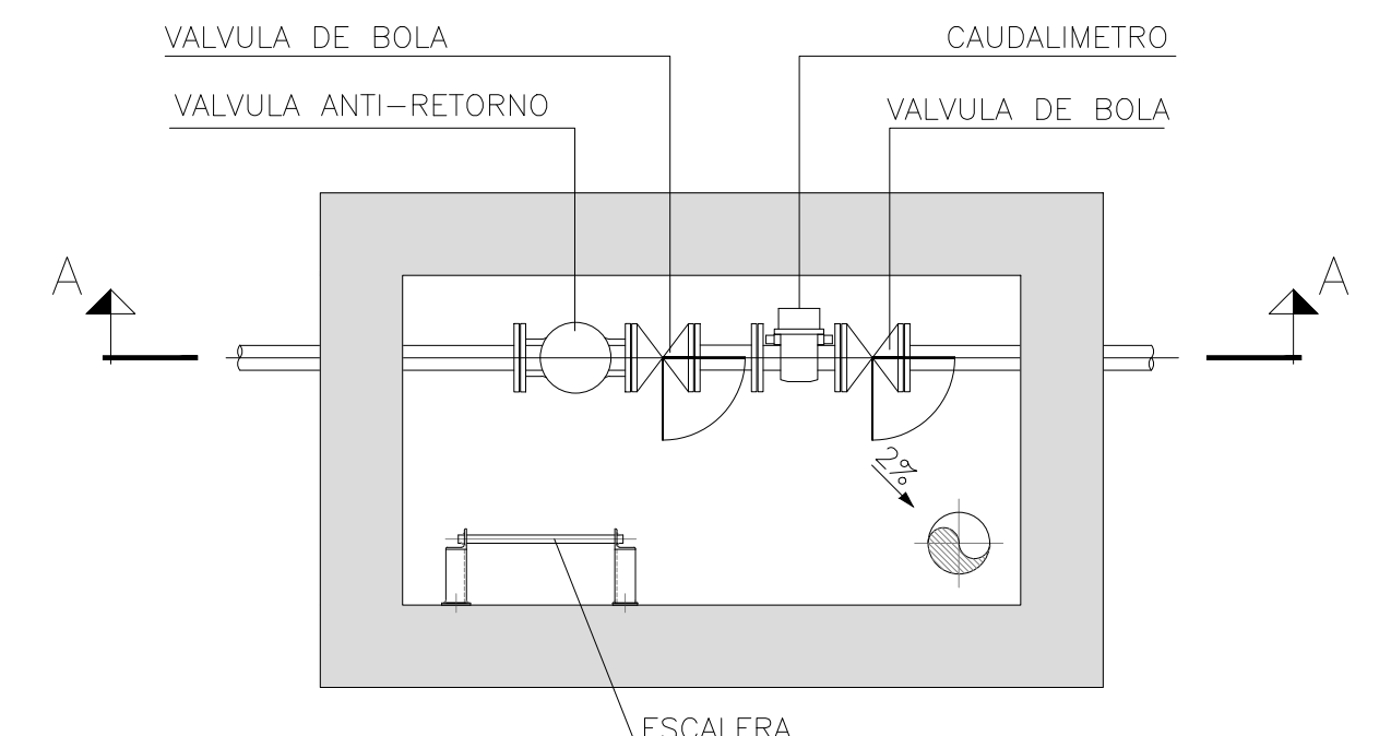
ARQUETA ACOMETIDA DETALLE TIPO ESCALA: S/E
